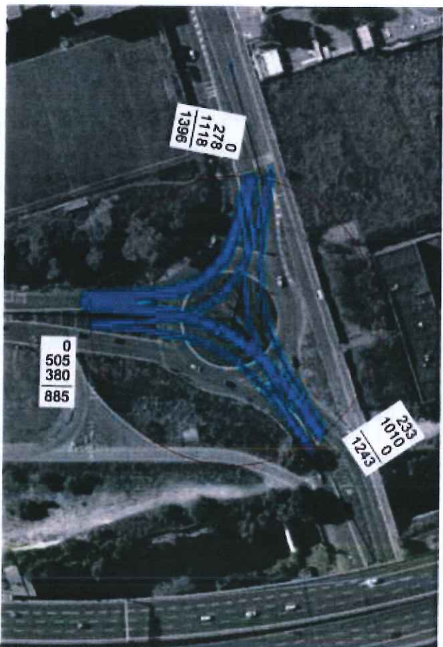
Figura 24 - Rotatoria 1 - Flussogramma in veicoli equivalenti relativo all'ora di punta della sera
