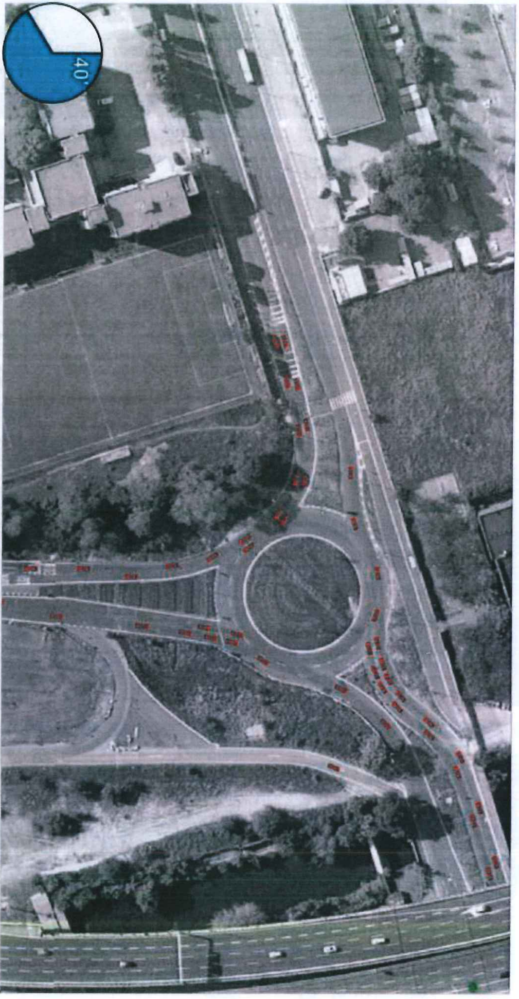
Figura 68 - ScENARIO SDF - Rotatoria 1 - Istantanea dopo 40 minuti di simulazione
