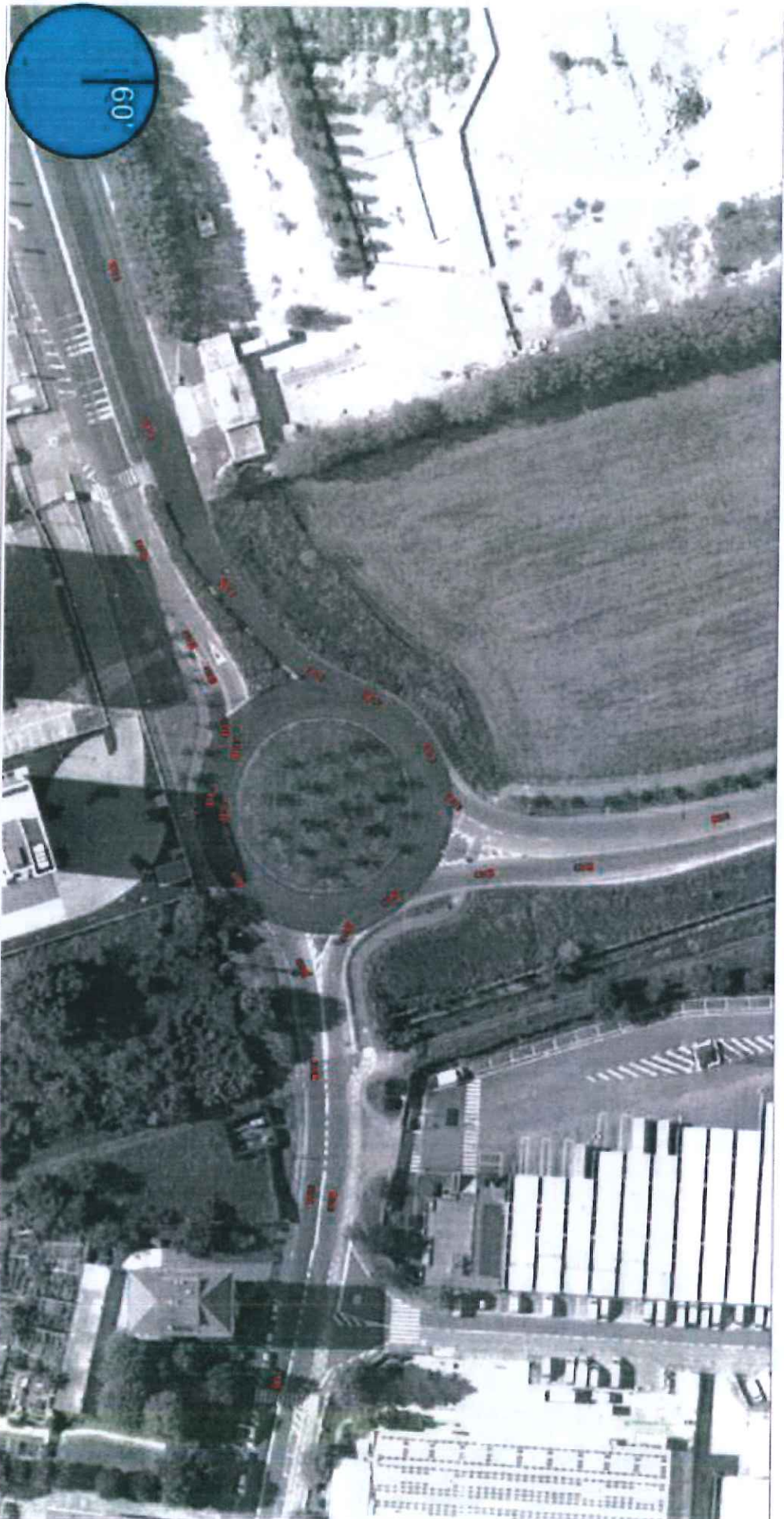
Figura 60 - Scenario SDF - Rotatoria 2 - Istantanea dopo 60 minuti di simulazione
