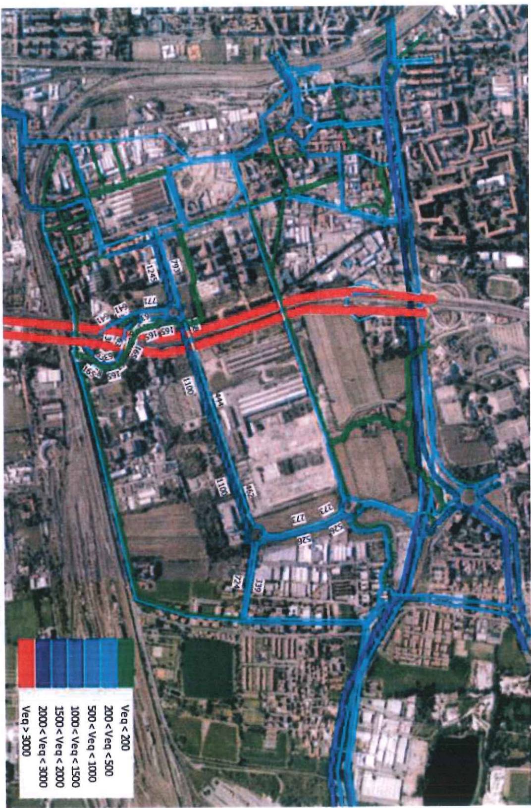
Figura 40 – Scenario di Riferimento ora di punta della sera – Flussogramma area di studio
