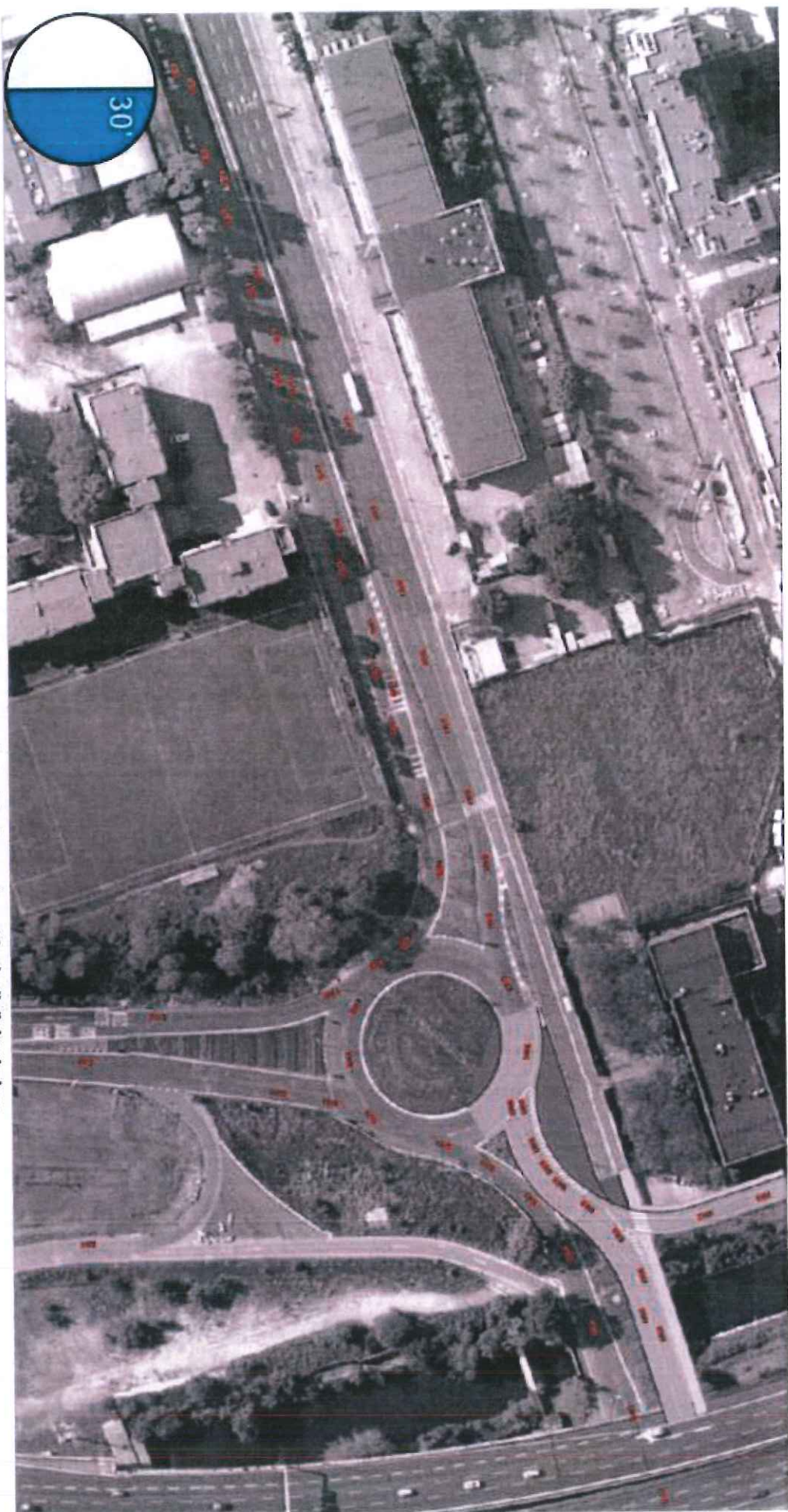
Figura 88 - Scenario di Intervento – Rotatoria 1 – Istantanea dopo 30 minuti di simulazione
