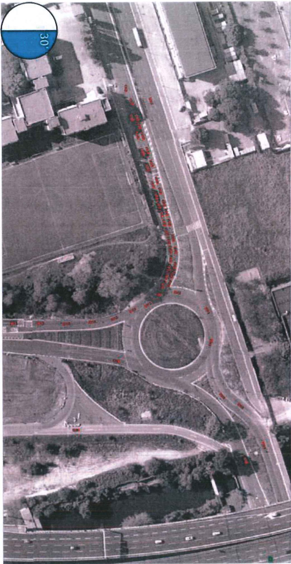
Figura 67 - Scenario SDF – Rotatoria 1 – Istantanea dopo 30 minuti di simulazione
