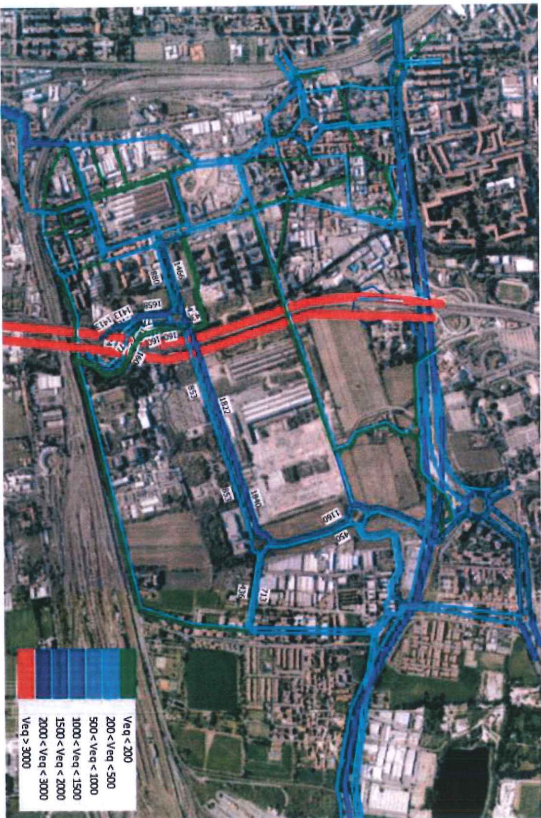
Figura 38 – Scenario di riferimento ora di punta del mattino – Flussogramma area di studio
