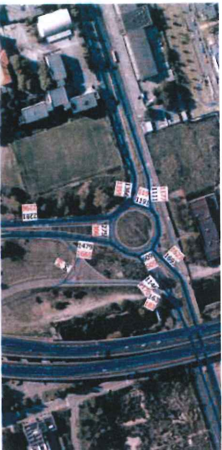
Figura 29 – Rotatoria 1: raffronto fra flussi rilevati (in rosso) e flussi simulati (in blu) – ora di punta del mattino
