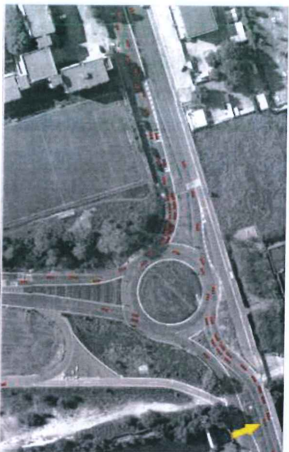
Figura 64 - Scenario SDF - Rotatoria 1 Rubattino/Svincoli AS1 - Accodamento massimo - Ramo 1C
