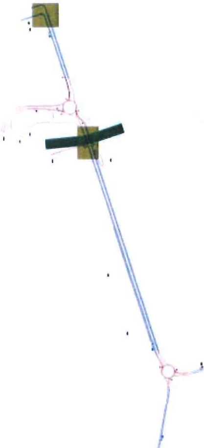
Figura 60 – Modello di microsimulazione –Scenario Attuale - Rete stradale
