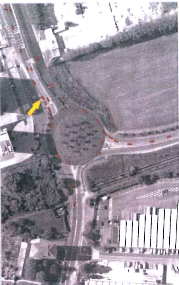
Figura 73 - Scenario SDF - Rotatoria 2 - Accodamento massimo - Ramo 2B
