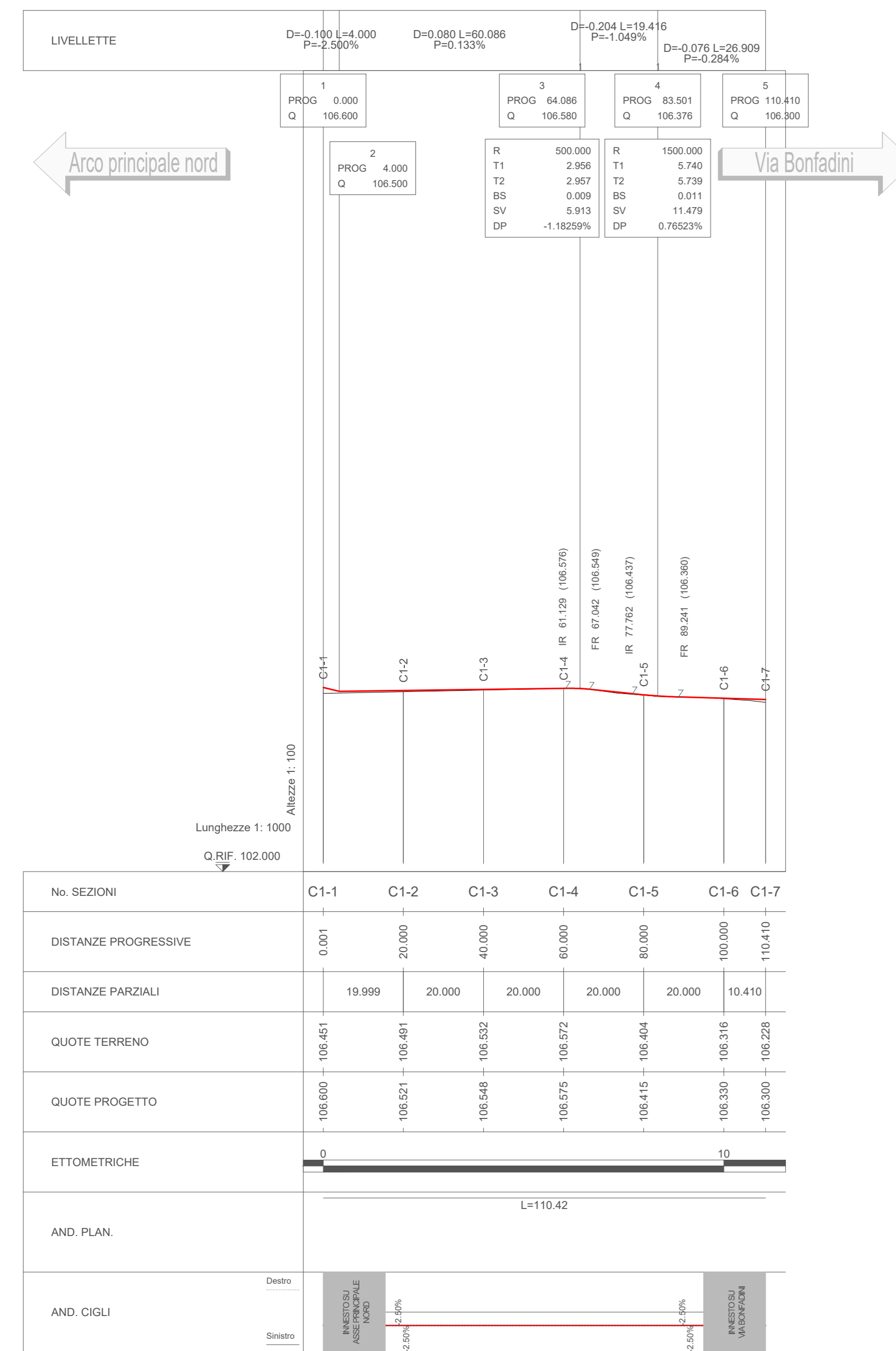
17 Profilo longitudinale - Collegamento 1 Scala 1:1000/100
