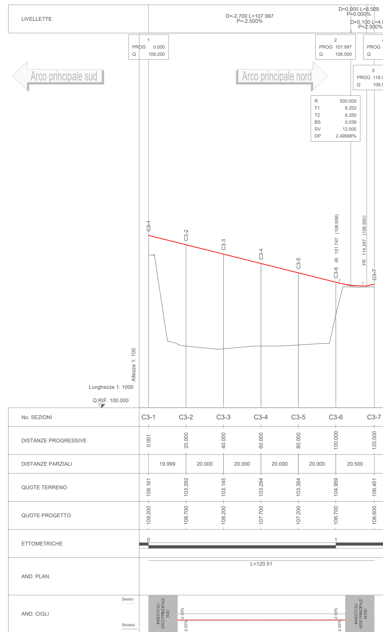
18 Profilo longitudinale - Collegamento 3 Scala 1:1000/100
