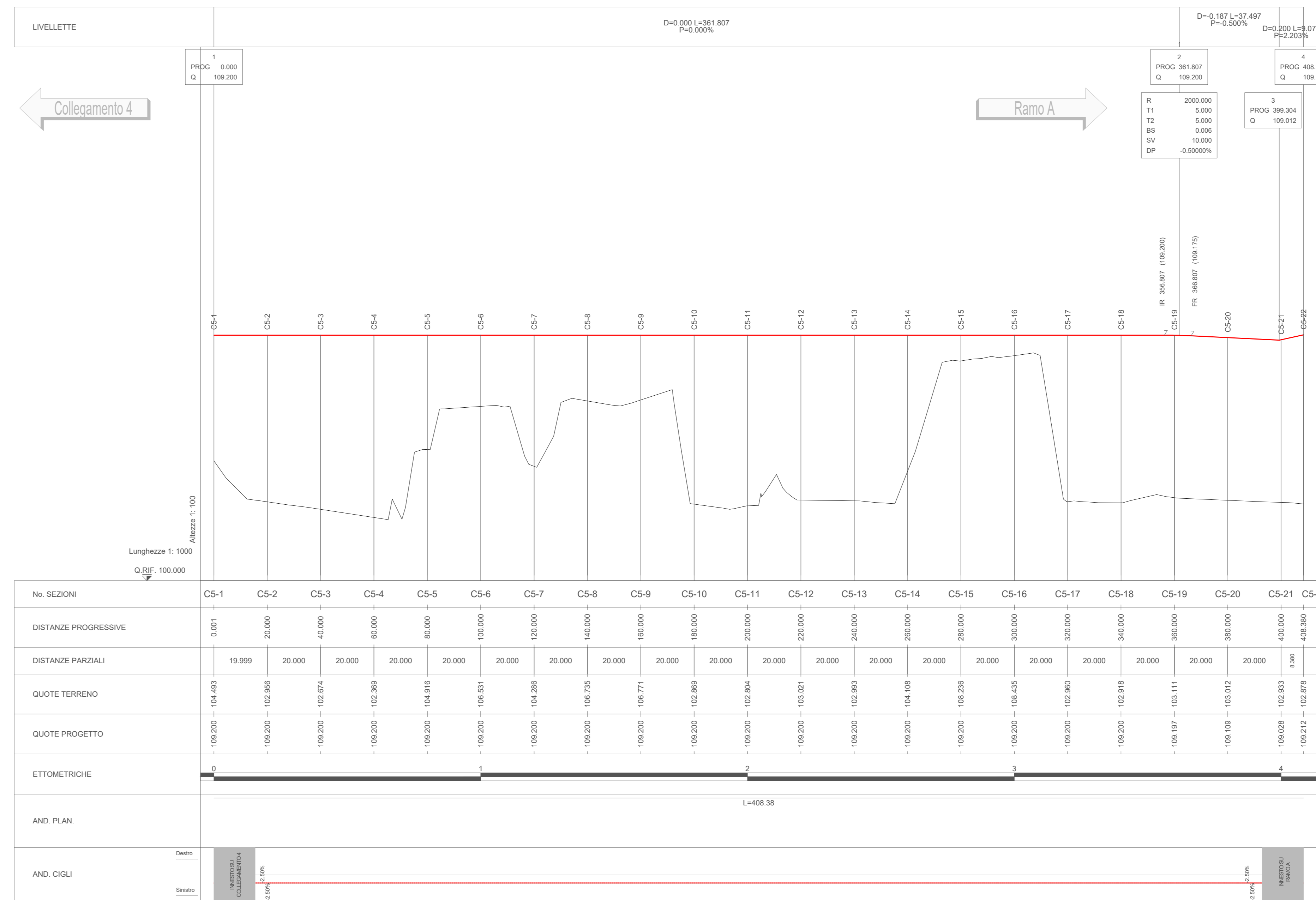
19 Profilo longitudinale - Collegamento 5 Scala 1:1000/100
