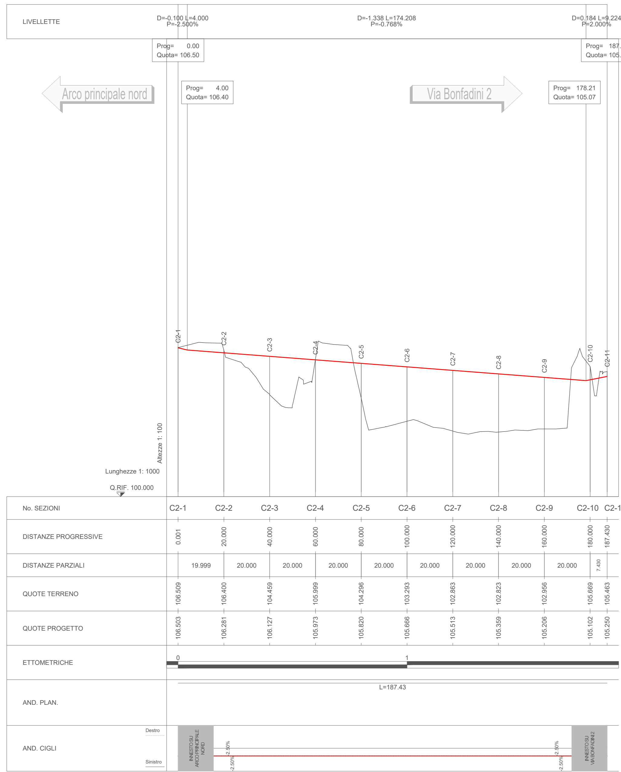
20 Profilo longitudinale - Collegamento 2 Scala 1:1000/100
